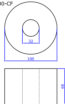
FI 9552 (Flange Isoladora)
