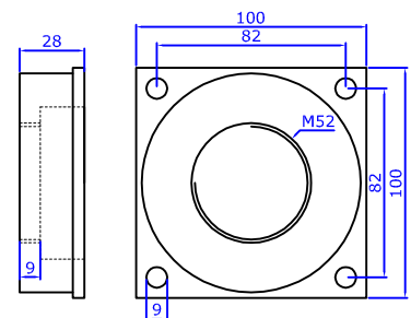
FI 9552 (Flange Isoladora)
